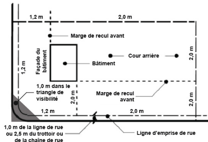
Figure 20 – Hauteur des clôtures et haies pour les lots d'angle
