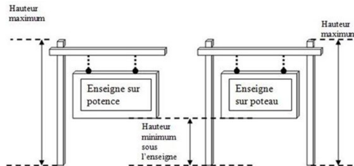
Figure 23 – Hauteur d'une enseigne sur poteau ou potence
