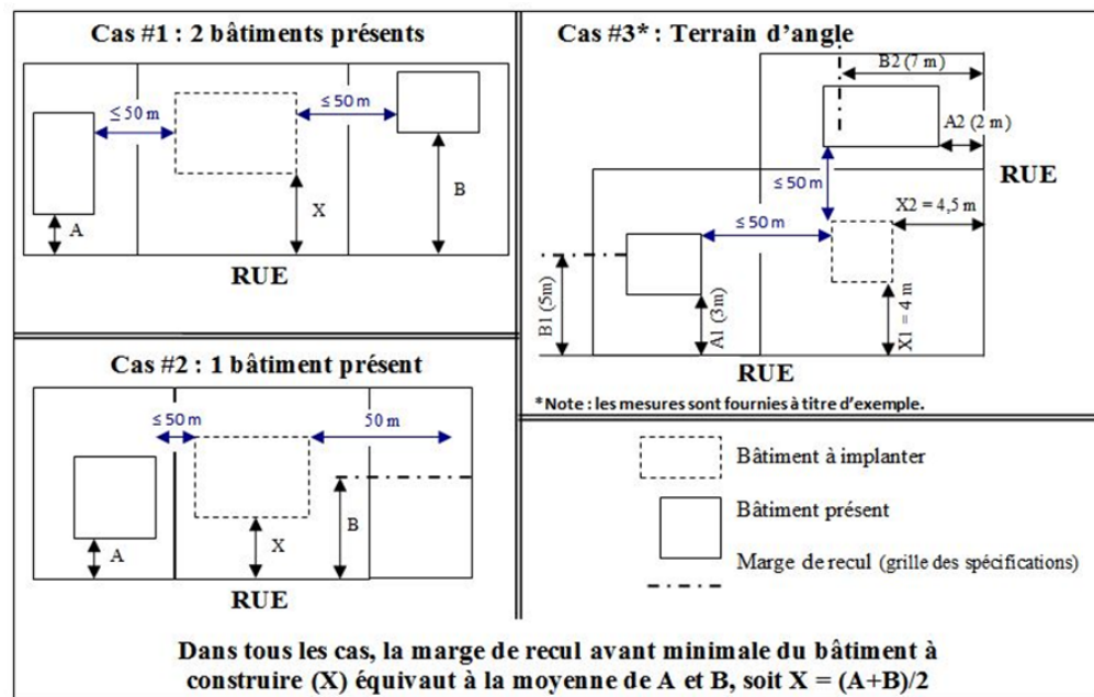
Figure 19 – Marge de recul avant dans les secteurs construits
