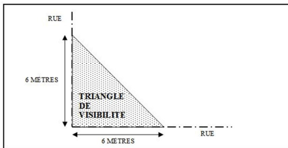
Figure 17 – Triangle de visibilité
