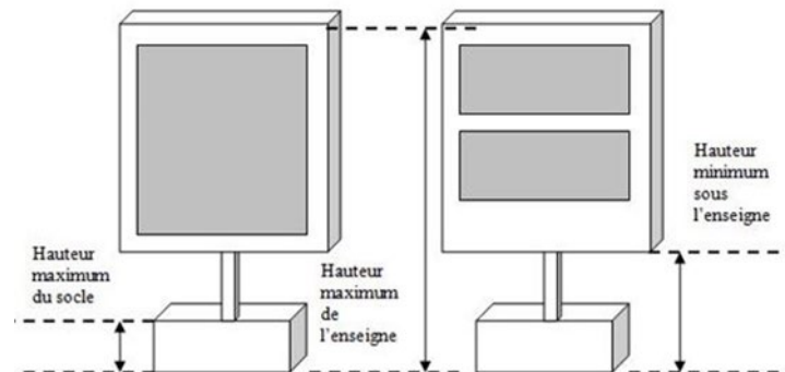
Figure 24 – Hauteur d'une enseigne sur socle
